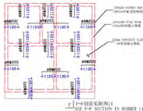
屋面板支座负筋配筋平面图
